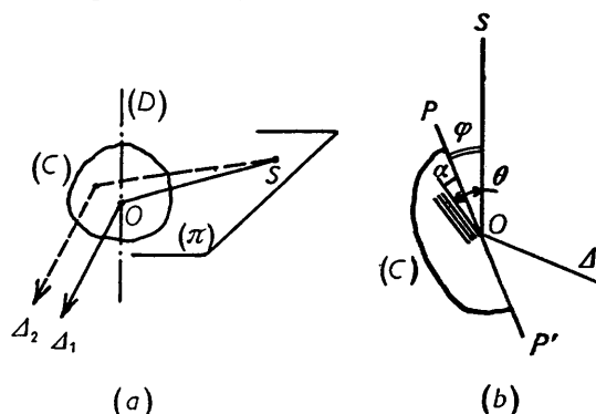
Fig. 1. Schéma expérimental. S , source de rayons X; ( D ) axe de rotation du cristal; ( Δ ) direction des faisceaux diffractés. (a) Cas général. (b) Cas des plans réticulaires ayant ( D ) comme axe de zone. Réflexion du rayon SO dans le plan ( π ) perpendiculaire à ( D ).
